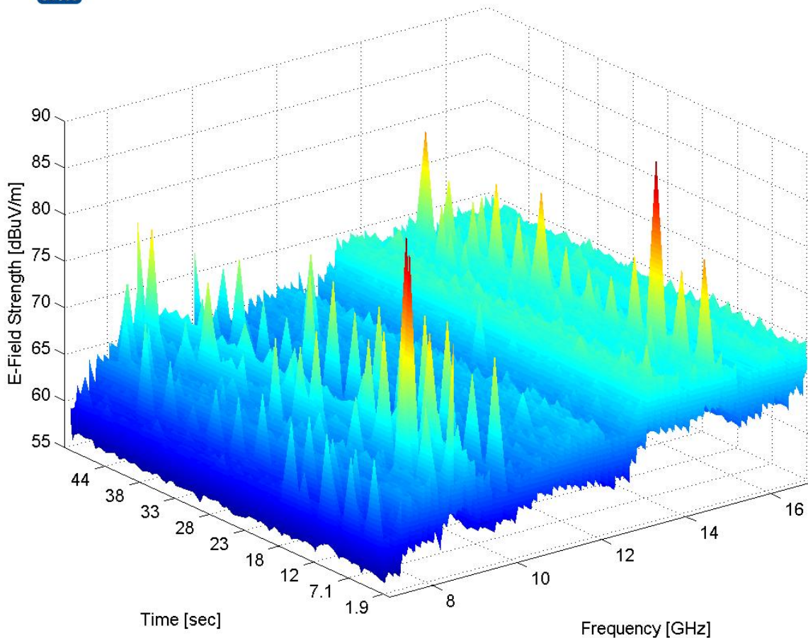
Fig. 2 – Real-time scanning von 6 bis 17 GHz, Messobjekt: Mikrowellenherd.
