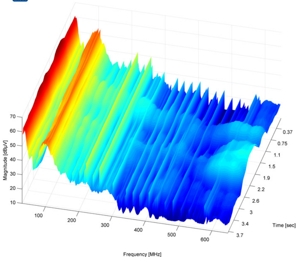
Fig. 2 – 645 MHz Echtzeitmessung 3D Darstellung
