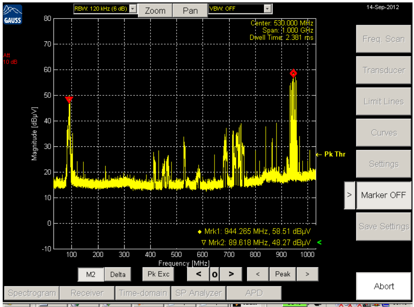
Fig. 1 – Spektralanalyzermodus
