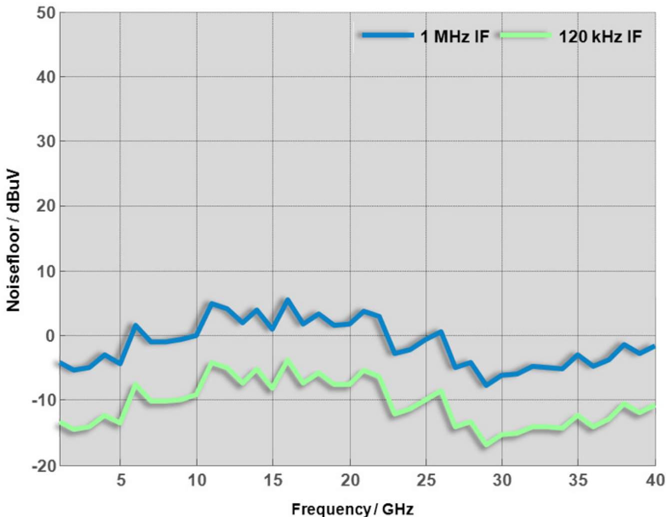
Fig. 1 – Niedrigstes Eigenrauschen bei 40 GHz
